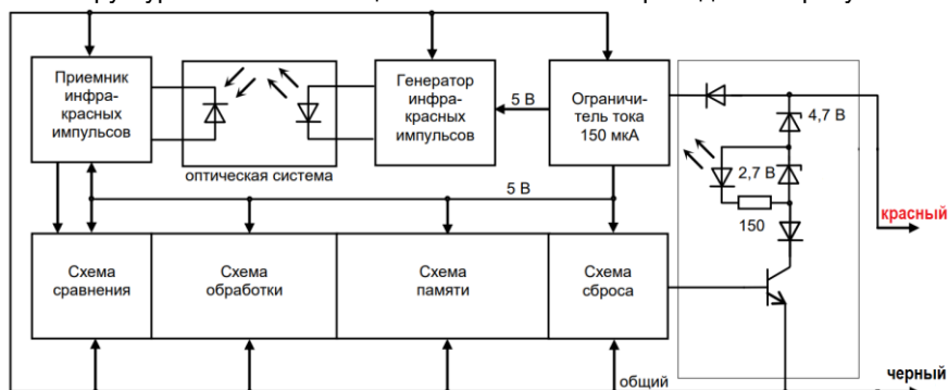
Рисунок 1 – Структурная схема извещателя ИП212-44Ех
