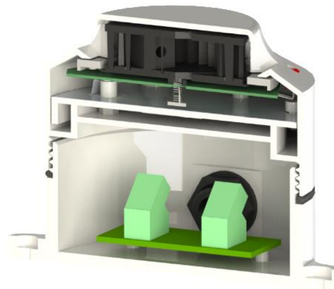
Рисунок 2 – Конструкция извещателей ИП212-44Ех в разрезе
