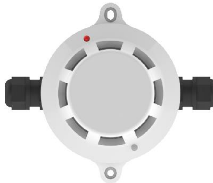
Рисунок 3 – Извещатели ИП212-44Ех (вид сверху)
