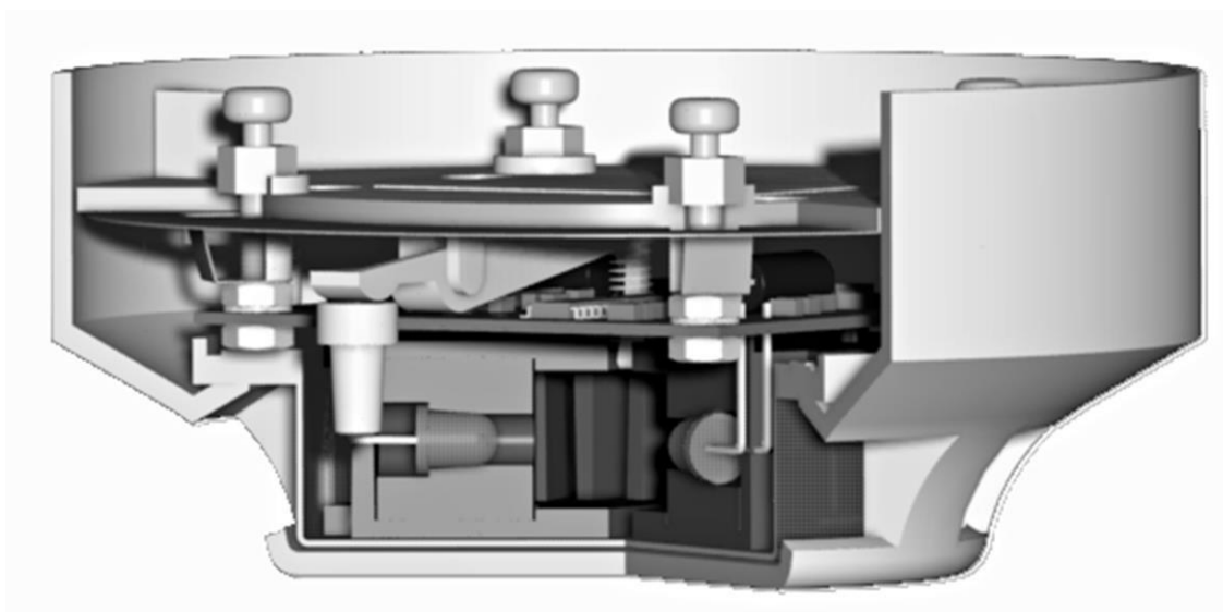
Рисунок 3 – Конструкция извещателей
